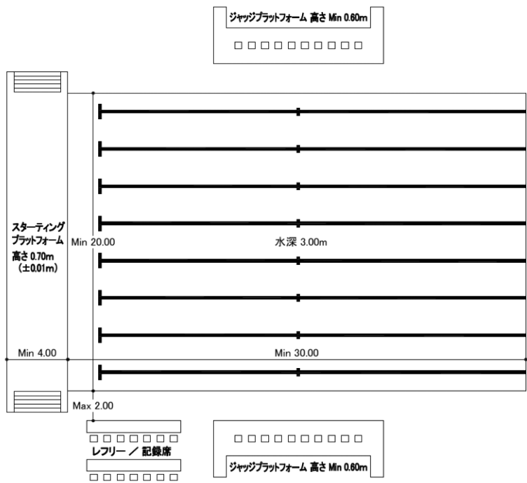
配置図
