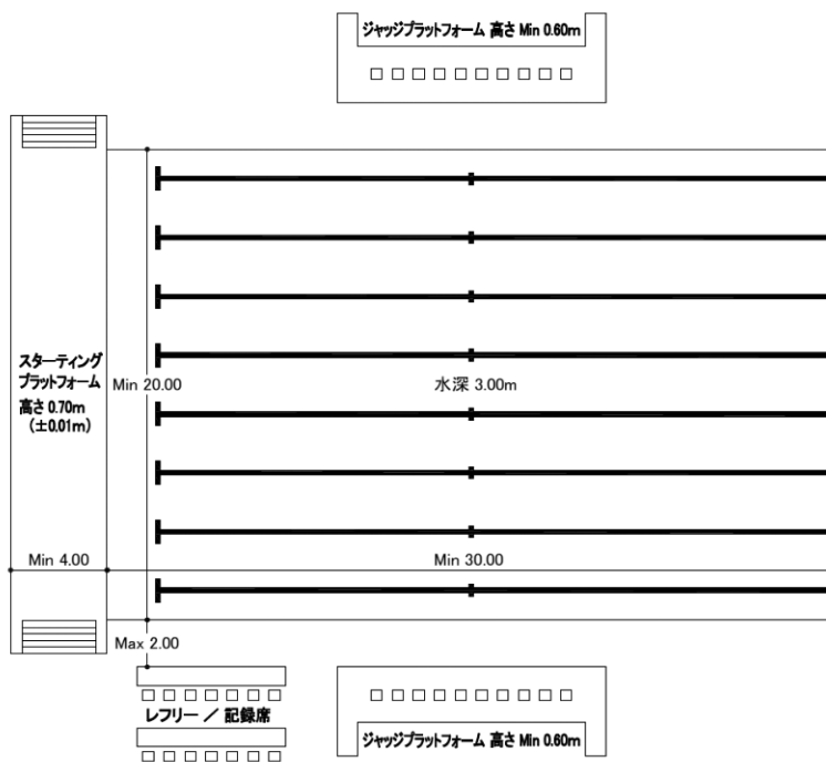
配置図
