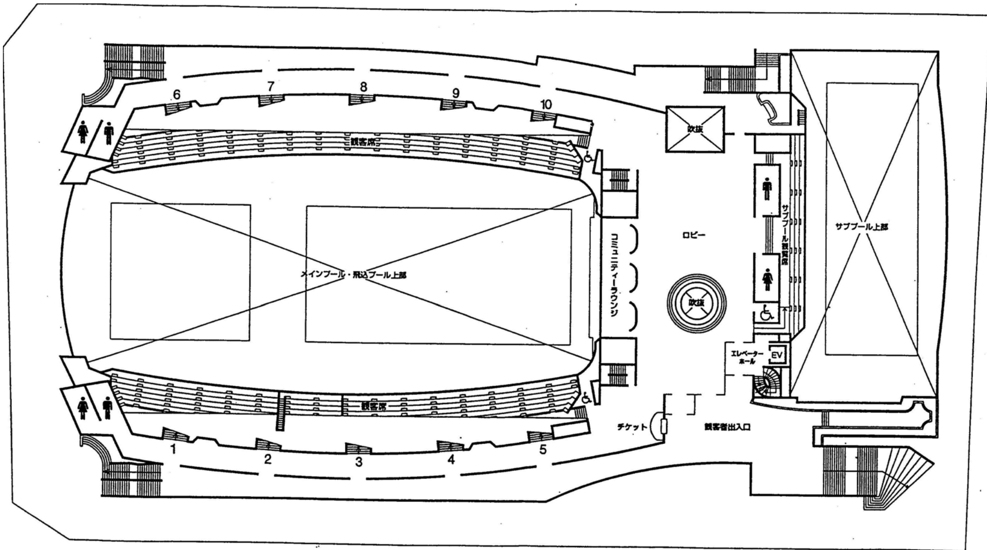
工務局建築設計部 設計図
