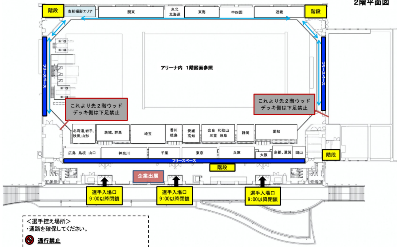
2階平面図
