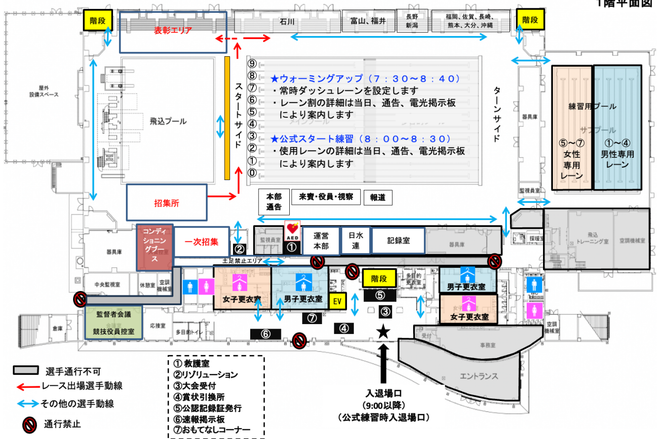
1階平面図
