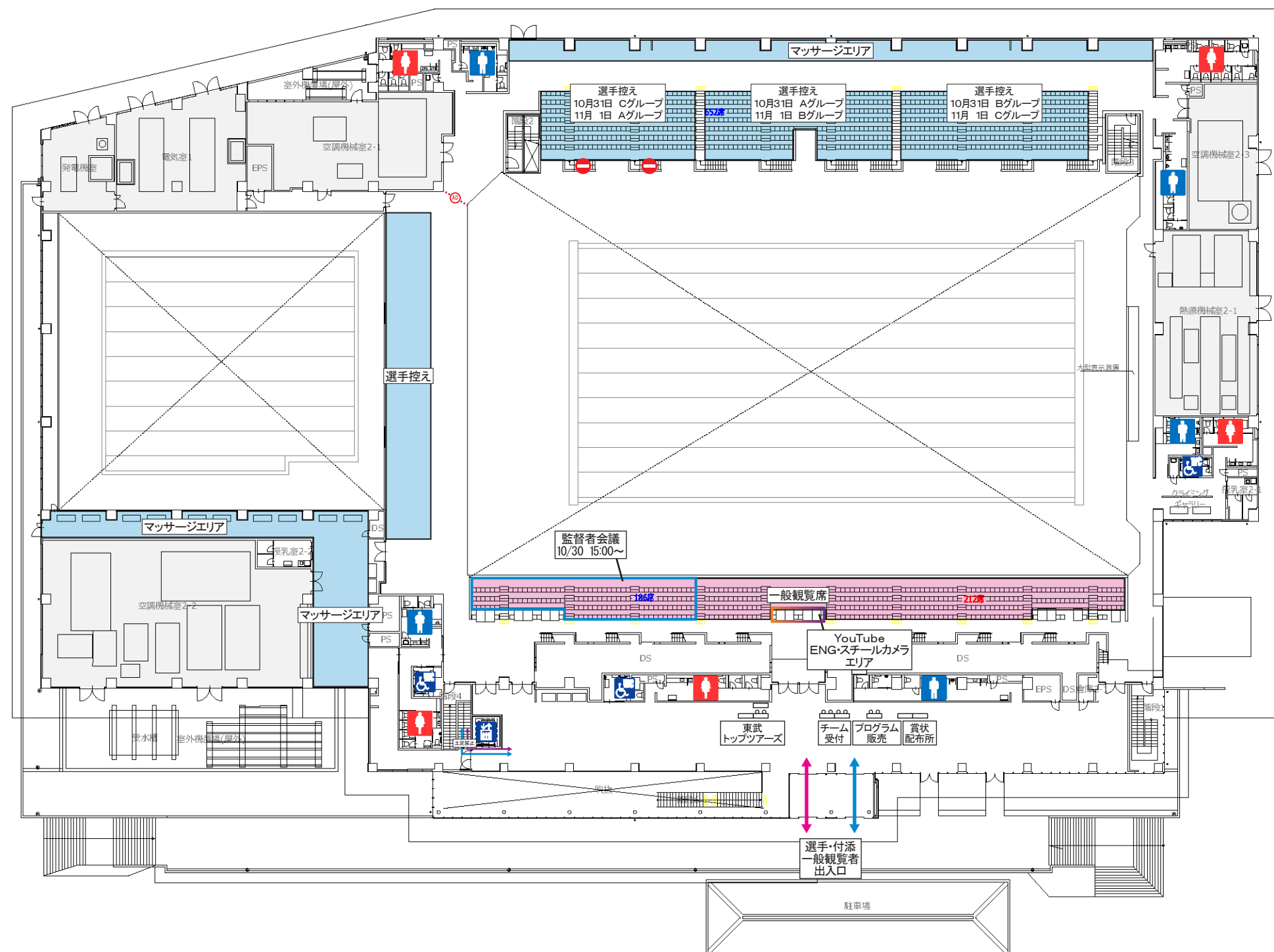
3階平面図
